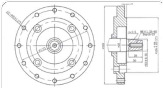
Albero - Shaft \varnothing 23 mm Flangia - Flange Mod.FL "L"
