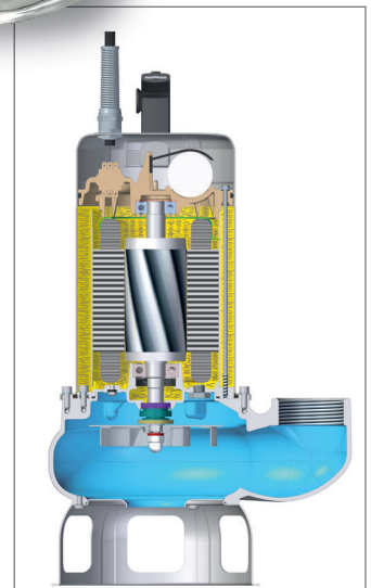
GIRANTE - IMPELLER
